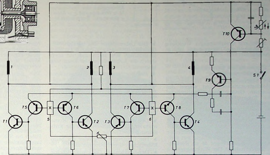
Bild 6. Schaltung des bürstenlosen Gleichstrommotors mit Hallgeneratoren und elektronischer Drehzahlregelung; 1, 2, 3, 4 Ständerwicklung, T1, T2, T3, T4 Leistungstransistoren, T5, T6, T7, T8 Vorstufentransistoren, 5, 6 Hallgeneratoren
