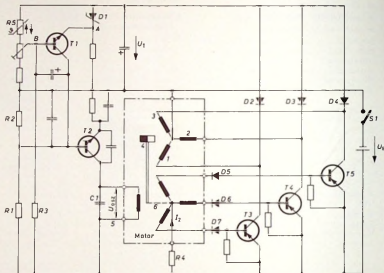
Bild 3. Aufbau des bürstenlosen Gleichstrommotors mit Hilfsfrequenz-Kommutator; 1, 2, 3 Ständerwicklung, 4 Magnetaußenläufer, 5 Ständerpaket, 6 Steuerkern, 7 Oszillatorspule, 8 Steuersegment, 9 Steuerspule
