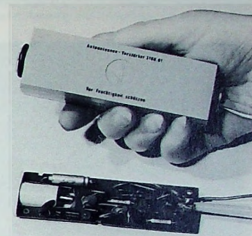
Kabelverstärker für Autoantennen (VEB Antennenwerke Bad Blankenburg)
