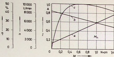
Bild 8. Kennlinien eines bürstenlosen Gleichstrommotors bei U_B = 21,5 \text{ V} Speisespannung; a Strom I in Abhängigkeit vom Drehmoment M , b Drehzahl n in Abhängigkeit vom Drehmoment M , c Wirkungsgrad \eta in Abhängigkeit vom Drehmoment M
