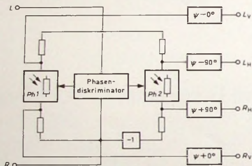
Bild 19. QS-Decoder mit Phasendiskriminator zur Erhöhung der Übersprechdämpfung
