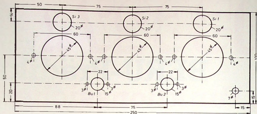
Bild 4. Bohrschema der Rückwand
