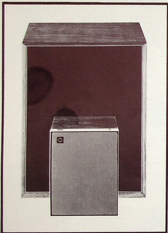
Die neue elektronische HiFi-Lautsprecherbox von Philips: RH 532 ELECTRONIC-MFB mit den Abmessungen 28 \times 38 \times 21 cm im Vergleich zu einer herkömmlichen 80-l-Box.
