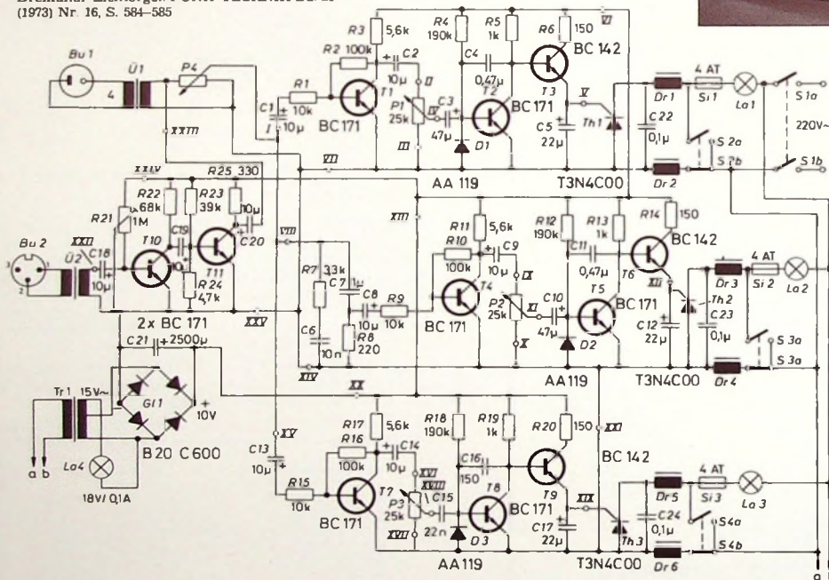
Bild 2. Gesamtschaltung der Lichtorgel mit Netzteil
